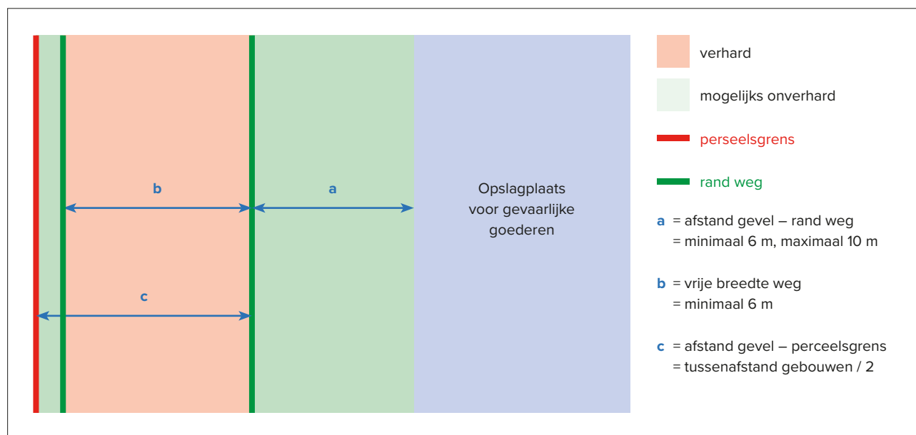
Figuur 2: Gevel zonder brandweerstand: minimumafstand gevel – rand weg is 4 m.
