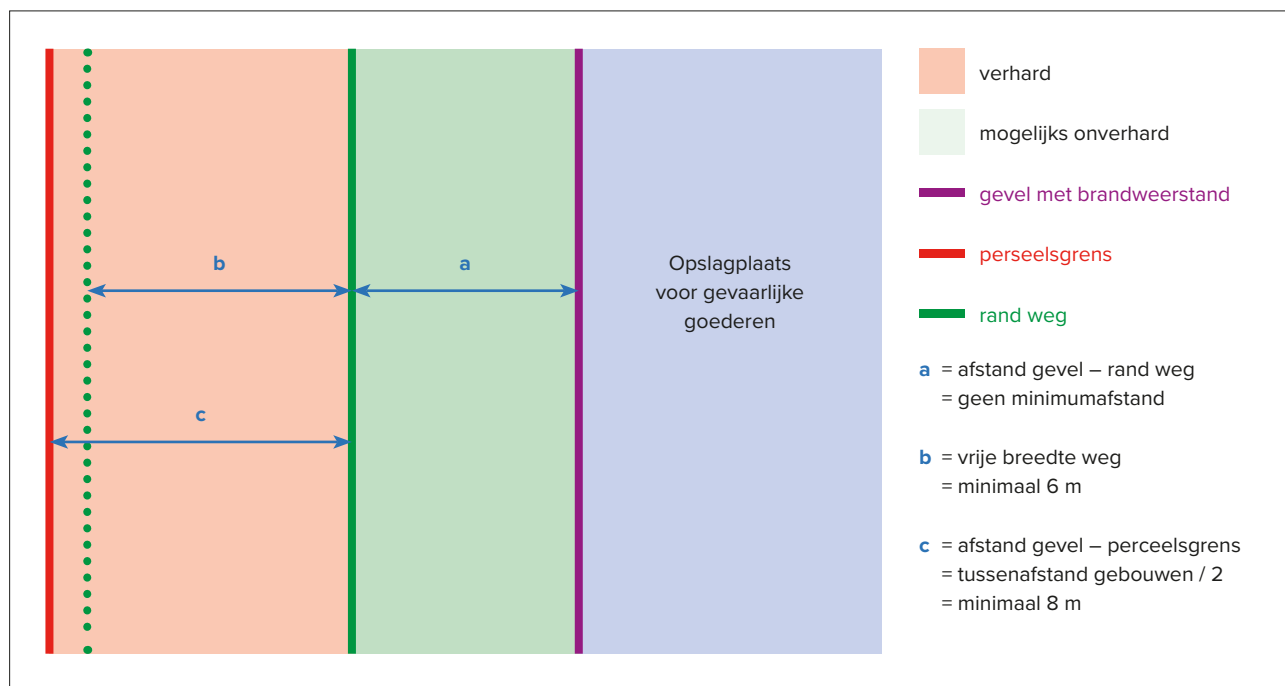
Figuur 3: Gevel met brandweerstand: geen minimumafstand gevel – rand weg.
